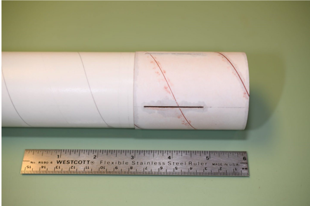
Photo 55: Fin Tab Slots
